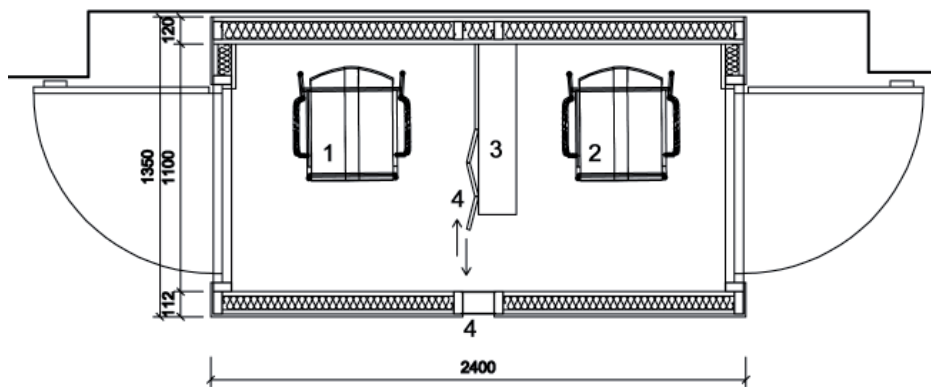
Půdorys zpovědnice (1-kněz, 2-kajícík, 3-kleátko, 4 shrnovací mřížka)
